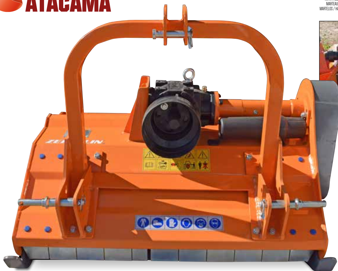
Tipo MZA. Arco Tripuntal
